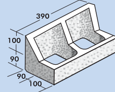
20.45 Header
