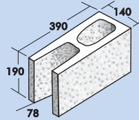
15.05 Open End
